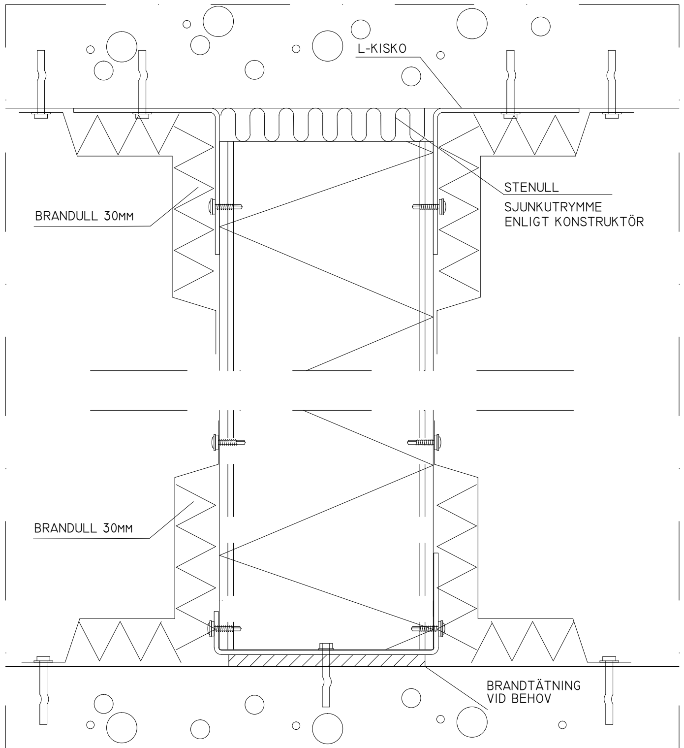
BRANDEDETALJ EI90-EI240
