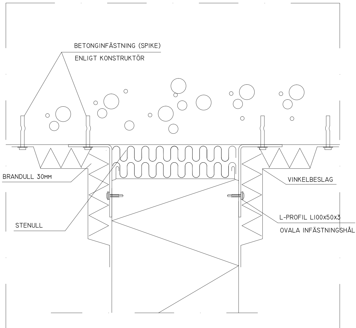
BRANDEDETALJ EI90-EI240
