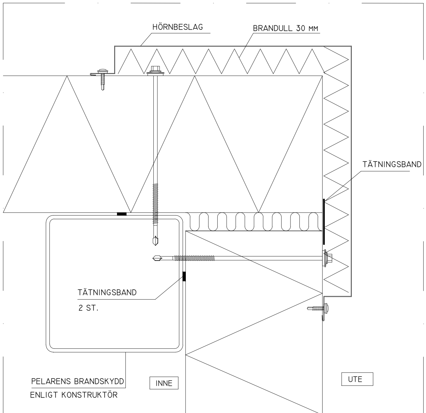
BRANDEDETALJ EI90-EI240
