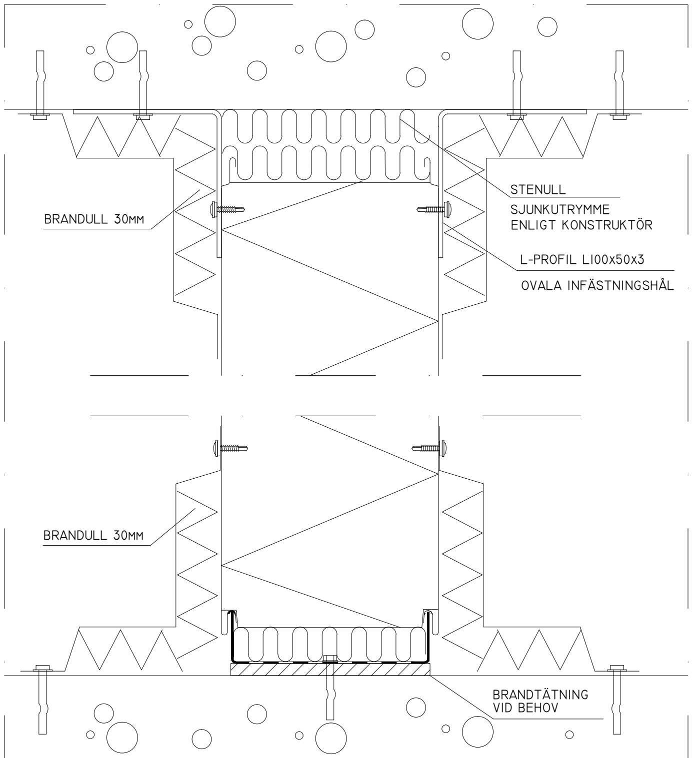
BRANDEDETALJ EI90-EI240
