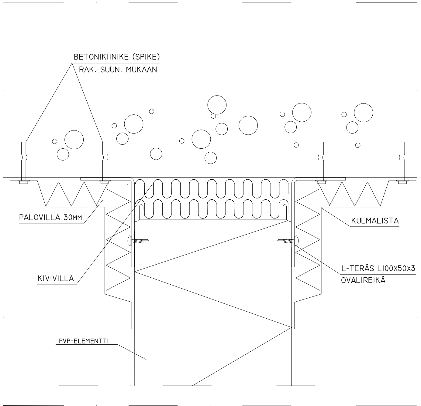
PALODELTAJI EI90-EI240
