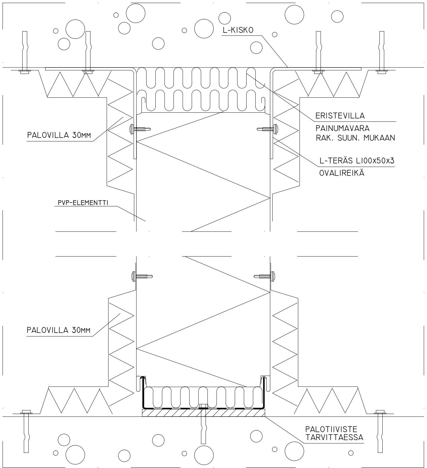
PALODELTAJI EI90-EI240
