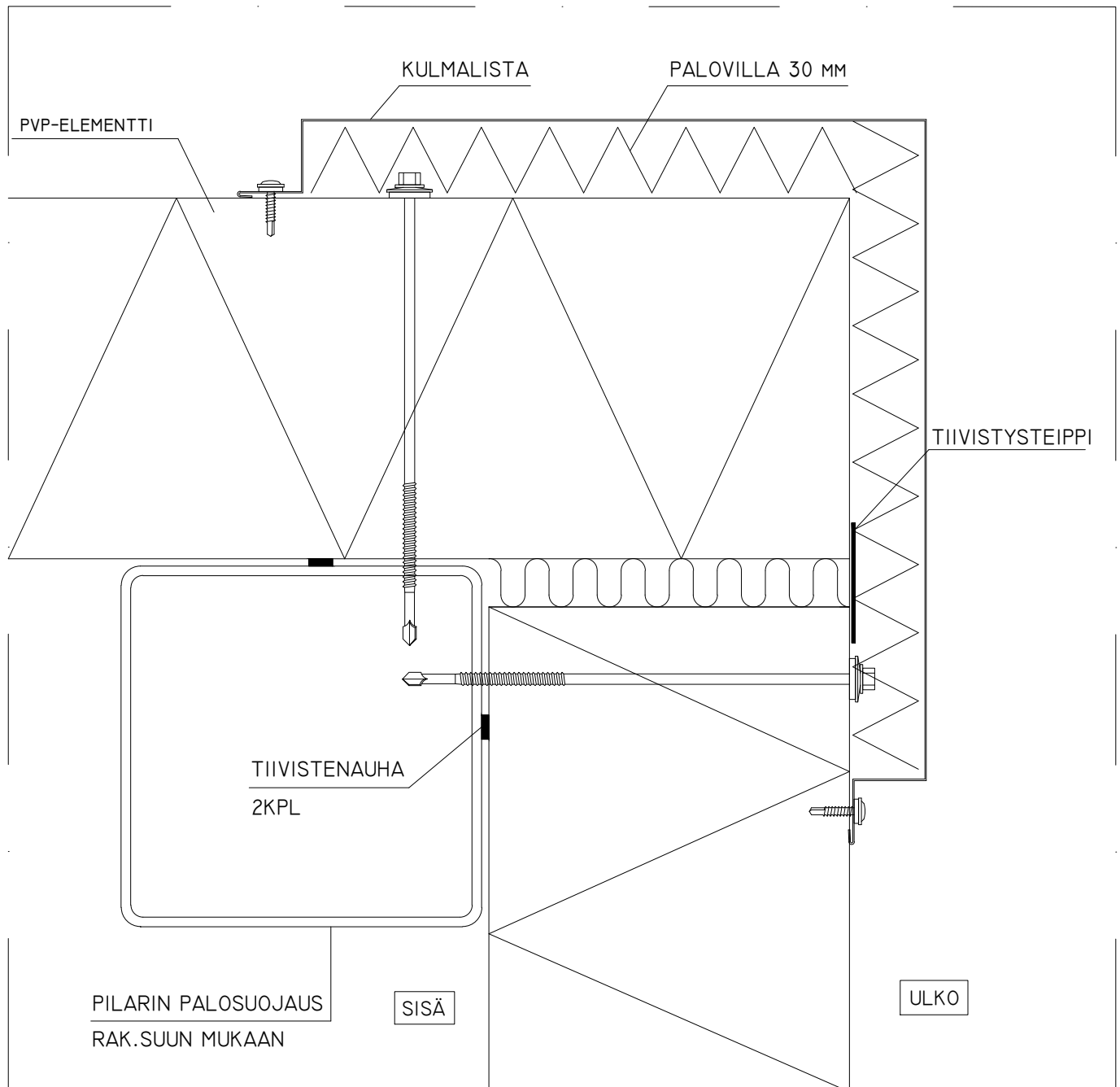
PALODELTAJI EI90-EI240
