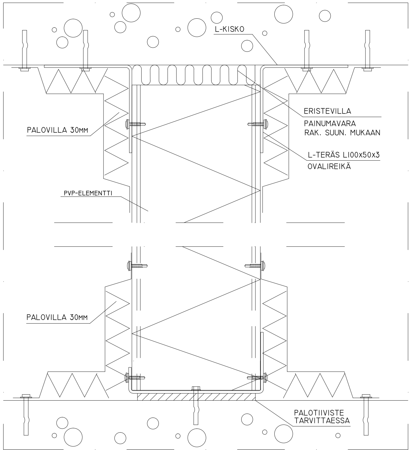
PALODELTAJI EI90-EI240
