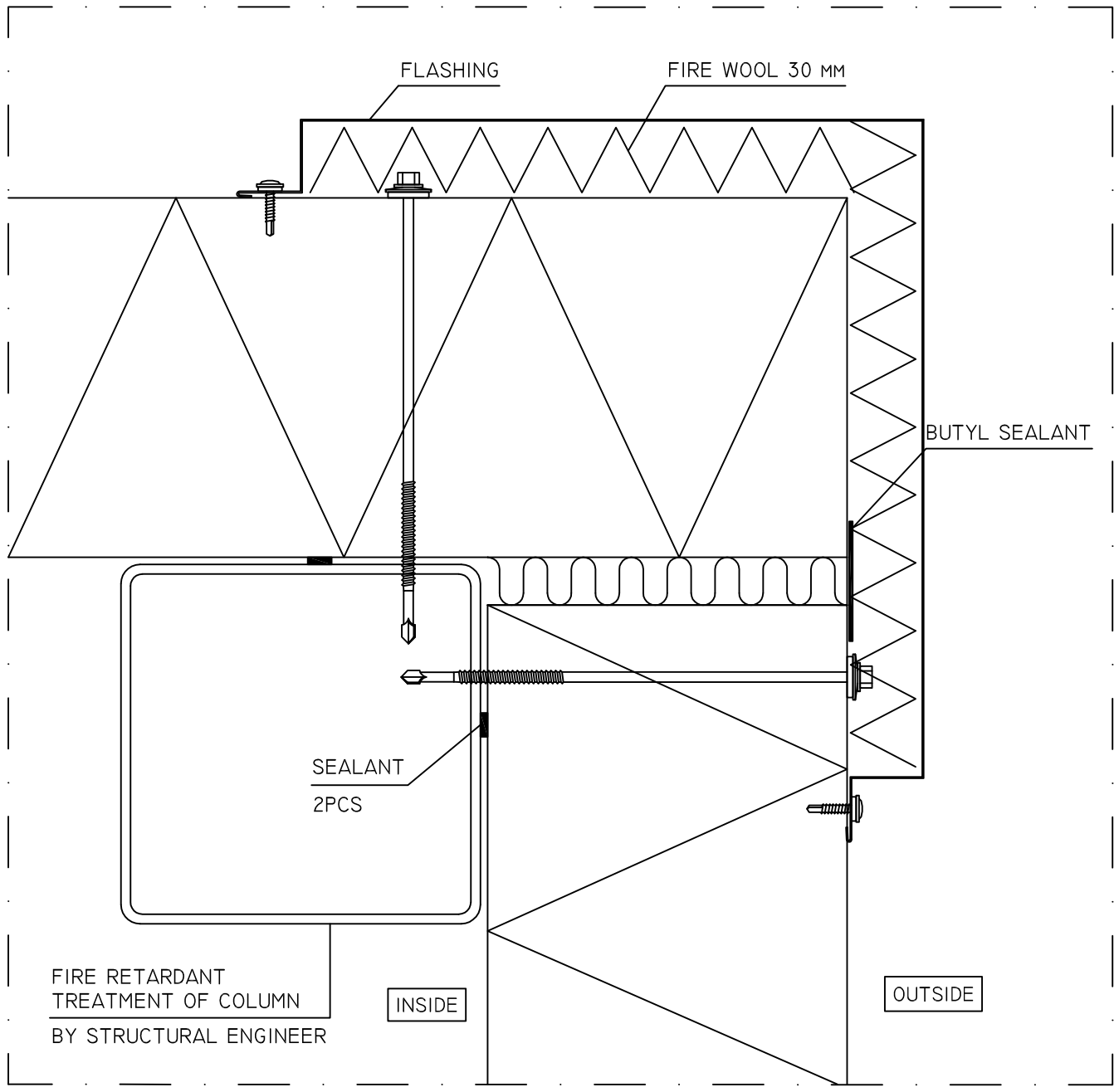
FIRE DETAIL E190-EI240
