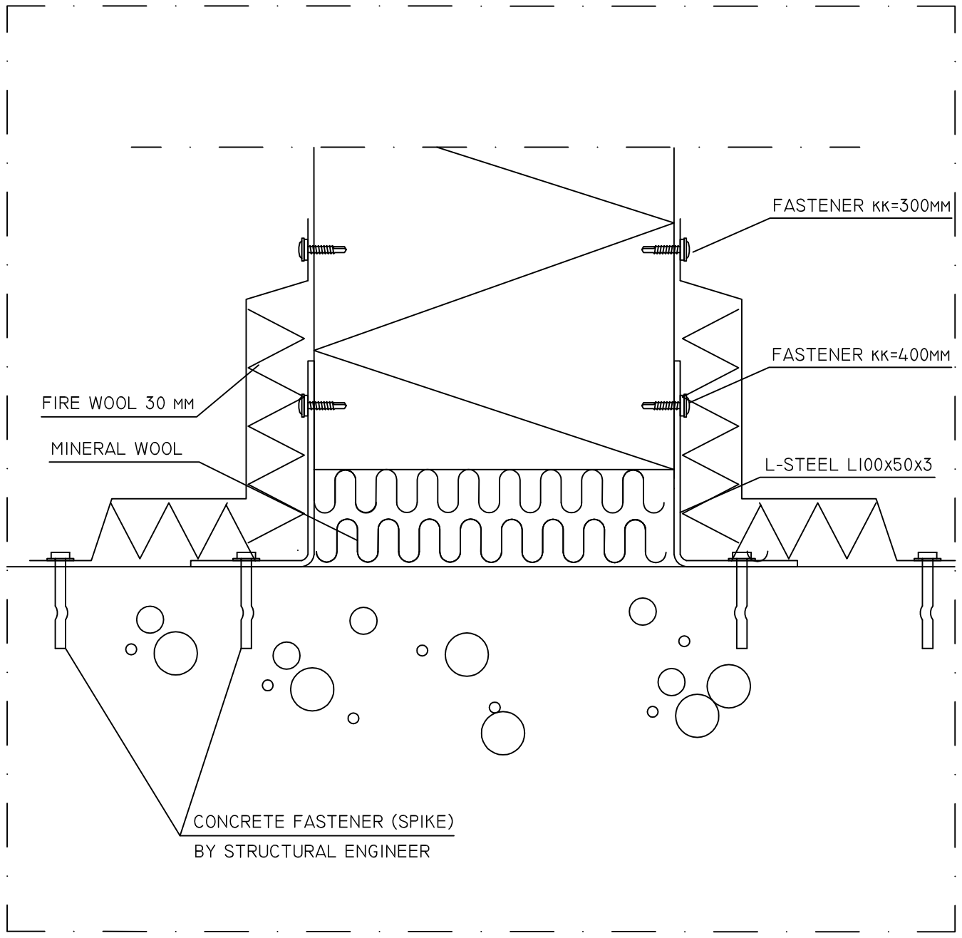
FIRE DETAIL E190-E1240
